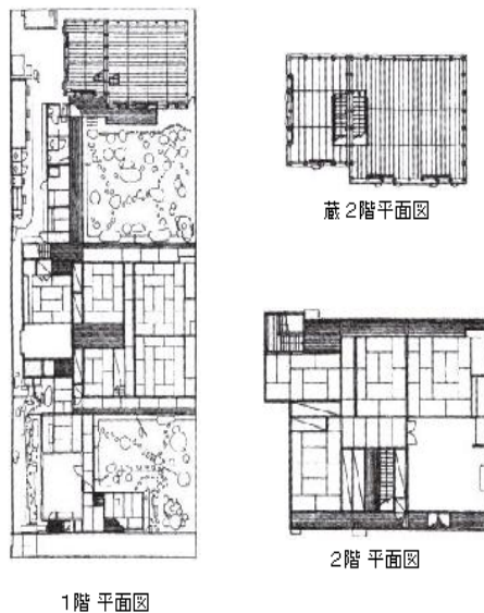
図2 紫織庵（大塀造）の平面図
